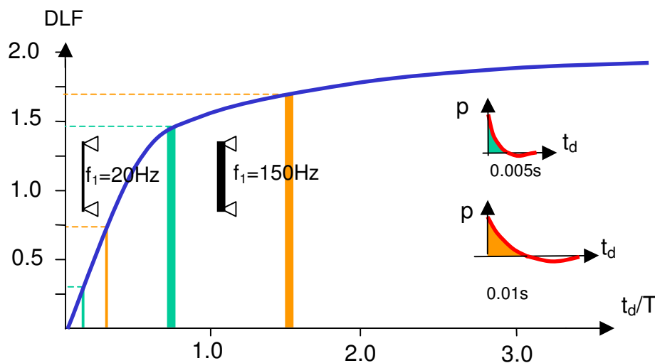
Bild 4: Tragwerkseinfluss
